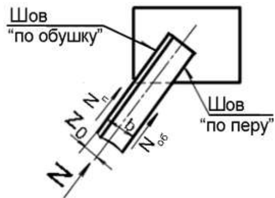
Рисунок 9 – Расчетная схема сварного узла
