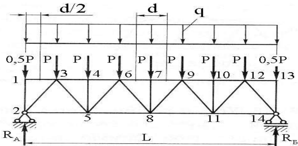
Рисунок 5 – Расчетная схема фермы
