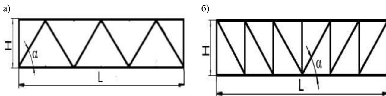
а – ферма с треугольной решеткой; б – ферма с раскосной решеткой; L – длина пролета фермы; H – высота фермы; \alpha – угол наклона раскосов
